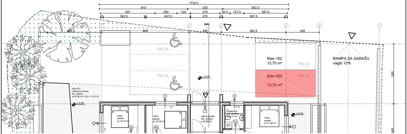
Pripadajući prostori - stan 002-V8 - PRIZEMLJE
