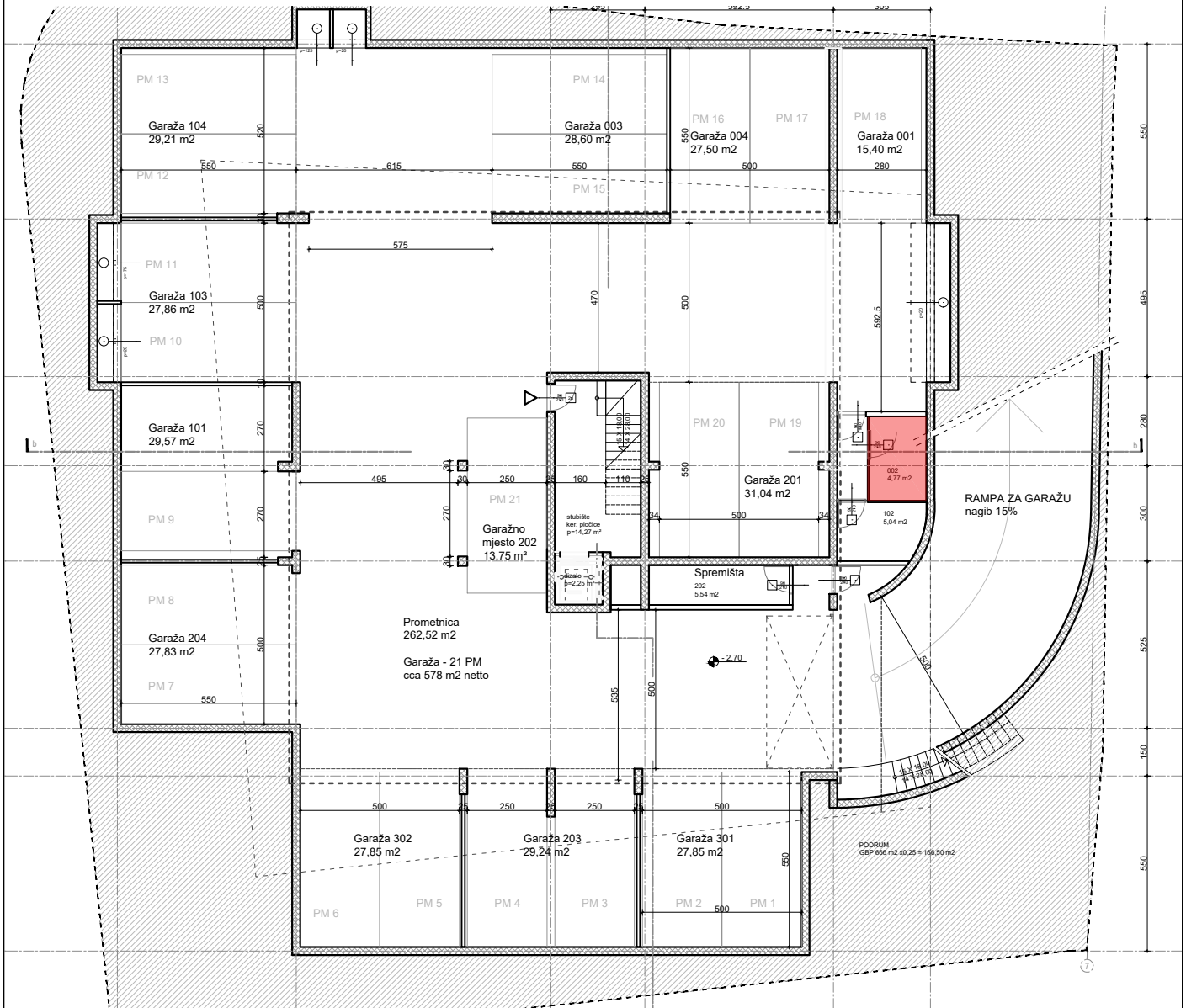
Pripadajući prostori - stan 002-V8 - GARAŽA
