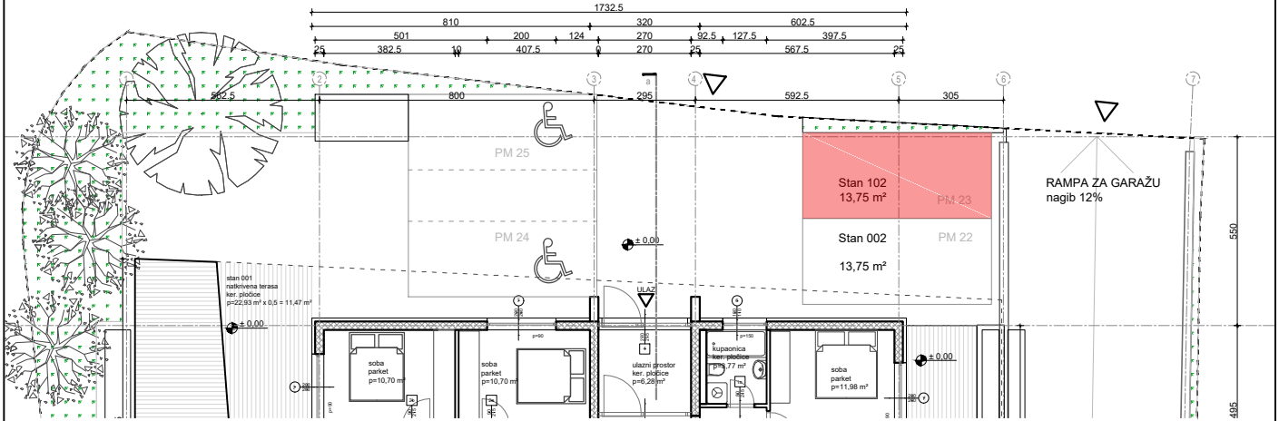
Pripadajući prostori - stan 102-V8 - PRIZEMLJE
