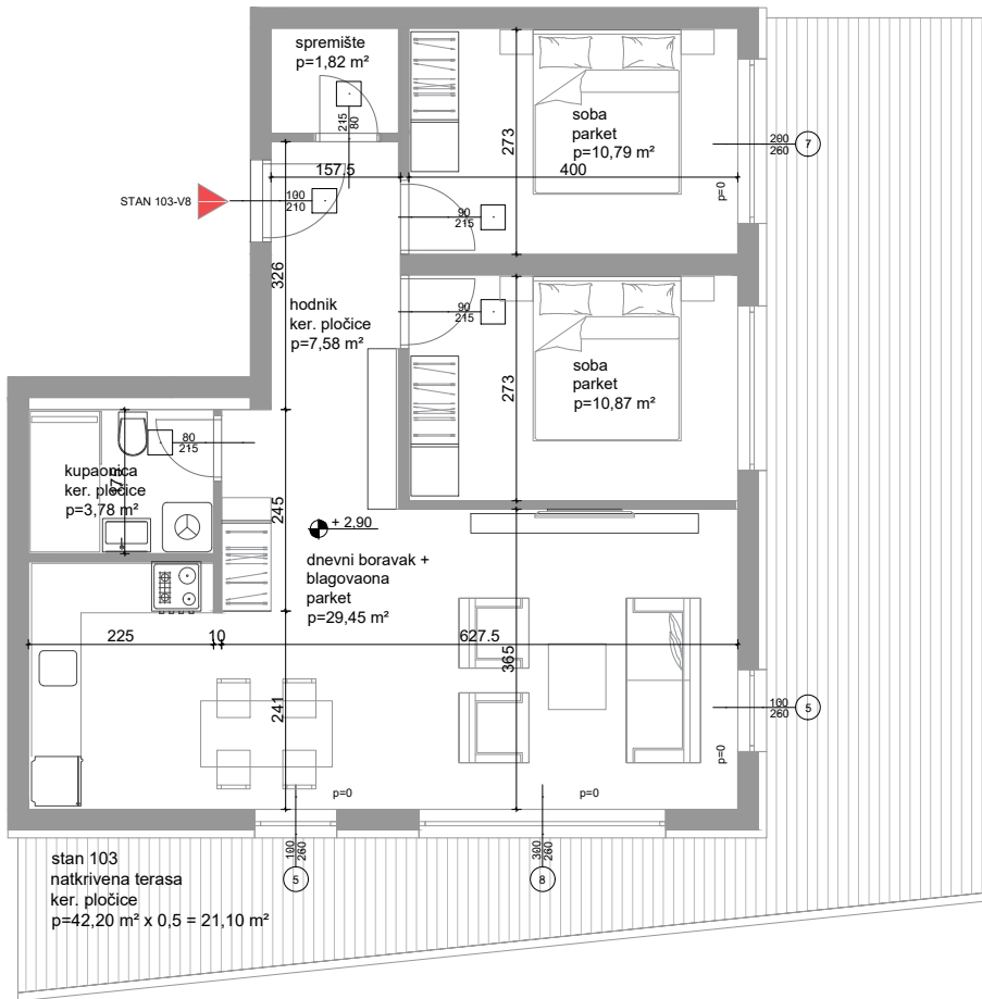
Tlocrt stana 103 - V8 - 1. KAT
