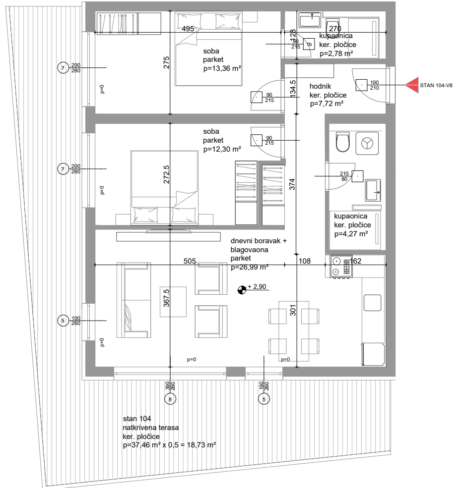
Tlocrt stana 104 - V8 - 1. KAT
