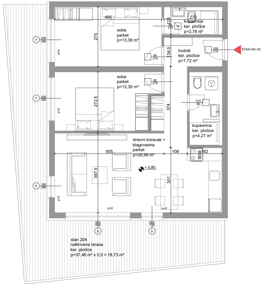
Tlocrt stana 204 - V8 - 2. KAT
